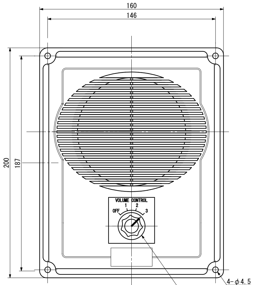
VOLUME CONTROL SW 音量調整器
