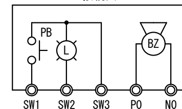
WIRING DIAGRAM 接続図
