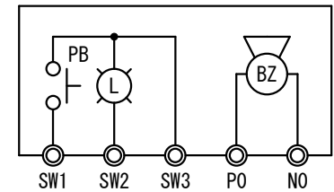
WIRING DIAGRAM 接続図
