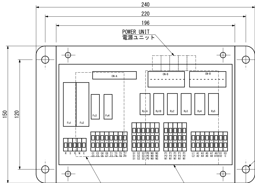
NOISE FILTER ノイズフィルタ RELAY TERMINAL P. C. B. リレー端子基板
