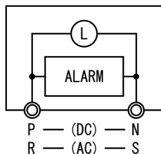
CONNECTION DIAGRAM 結線図
