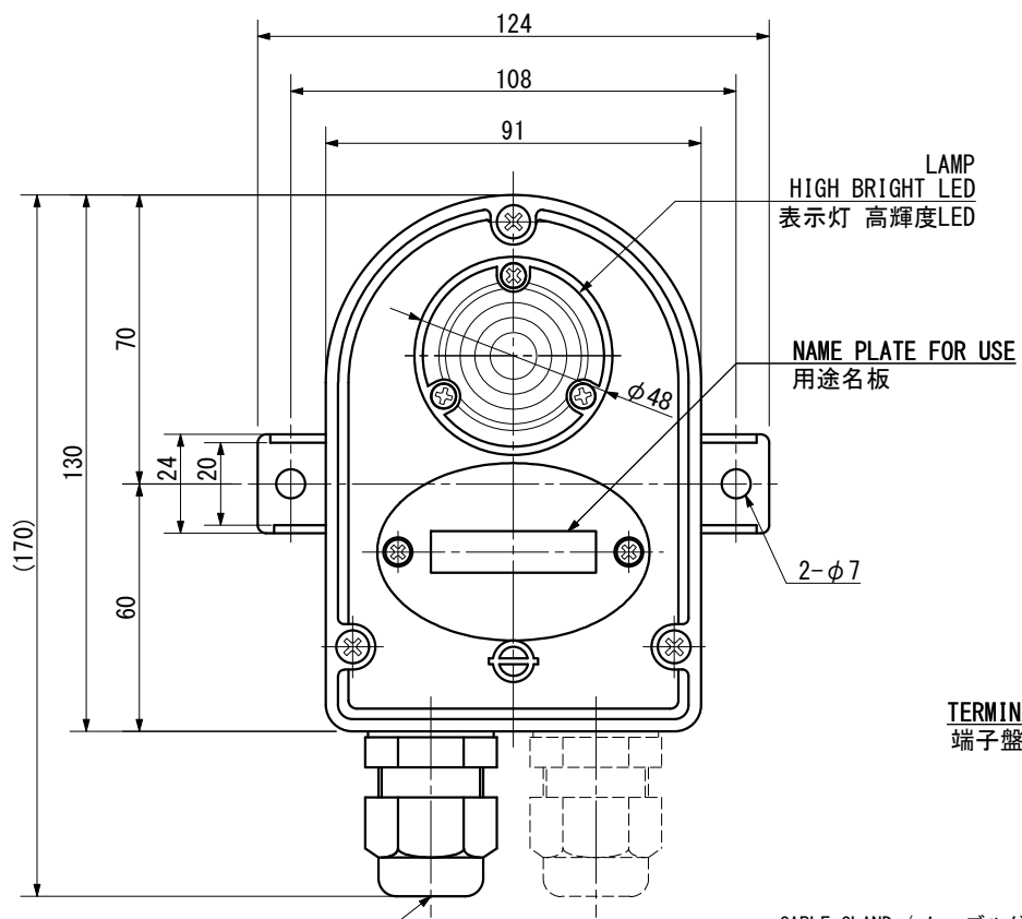
CABLE GLAND / ケーブルグランド
