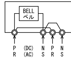
CONNECTION DIAGRAM 結線図
